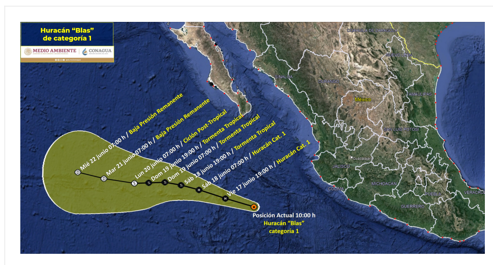
Trayectoria pronóstico del Huracán "Blas" Categoría 1.
